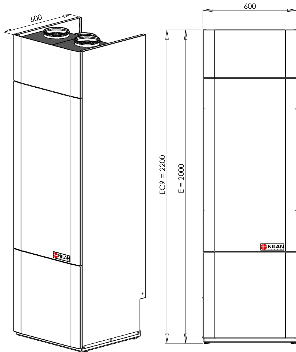
Nilan E-sarja mittakuva
